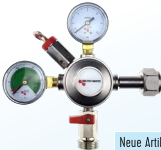
Druckminderer Einleitig mit Flascheninhaltsmanometer
